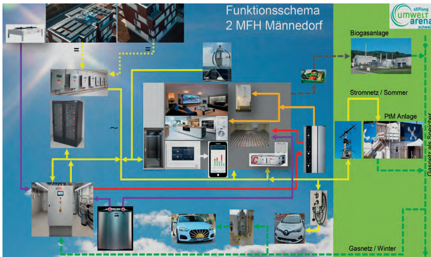
■ Funktionsschema der beiden Mehrfamilienhäuser in Männedorf. (Quelle: Umweltarena)
